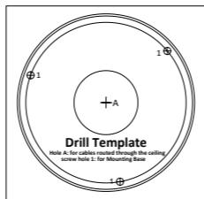
Рисунок 2-4 Шаблон крепления
