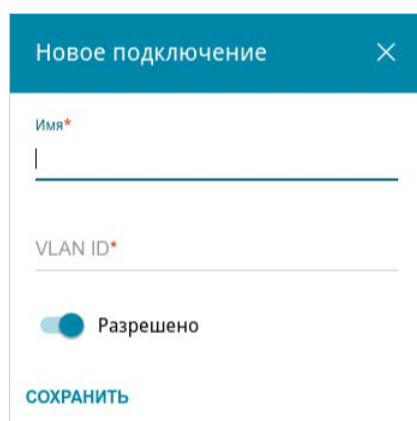
Рисунок 60. Добавление подключения.
