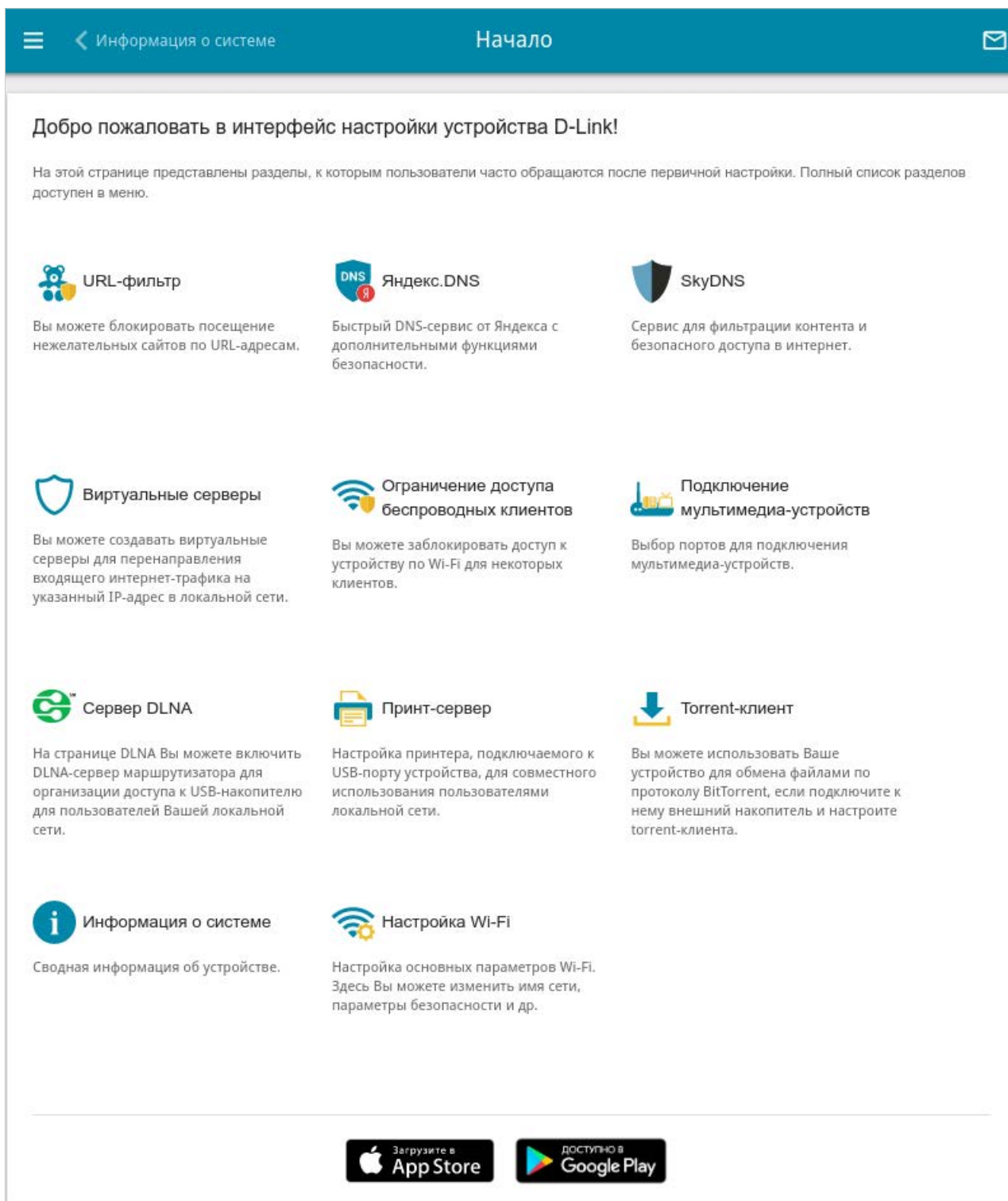
Рисунок 26. Страница Начало .
