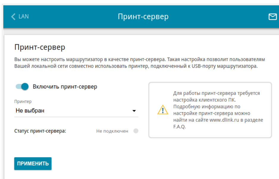
Рисунок 143. Страница Принт-сервер .
