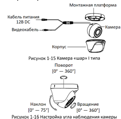
Рисунок 1-16 Настройка угла наблюдения камеры
