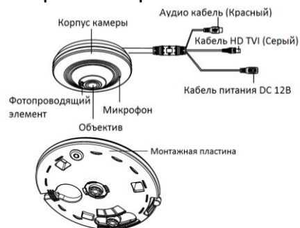
Рисунок 1-28 Панорамная камера
